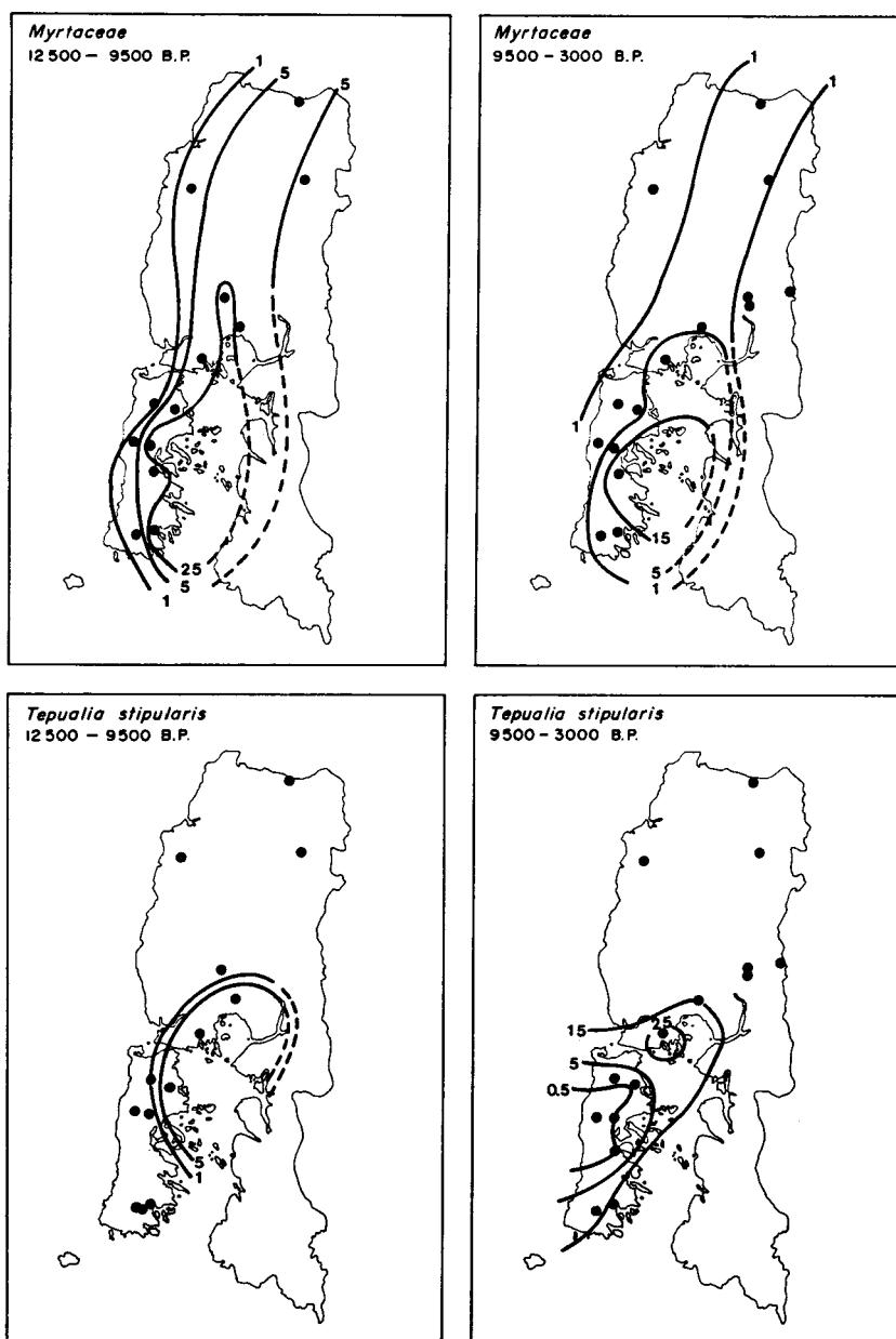
Fig. 3: Líneas isopolen para las Myrtaceae y Tepualia stipularis . Isopollen lines for Myrtaceae and Tepualia stipularis .
