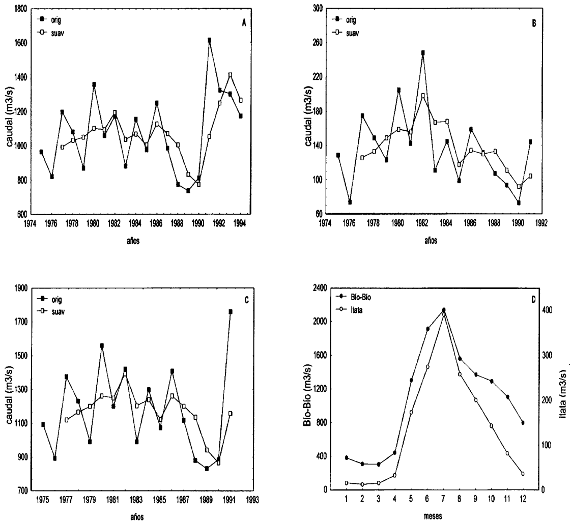
Fig. 2: Caudal medio anual (m 3 /s) de (a) río Bío-Bío durante el período 1975-1994, (b) río Itata durante el período 1975-1991, (c) índice \beta durante el período 1977-1991, y (d) señal mensual histórica del caudal de los ríos Bío-Bío e Itata calculada en base a 18 años y 15 años de información respectivamente. Serie de tiempo original (orig) y suavizada (suav).
