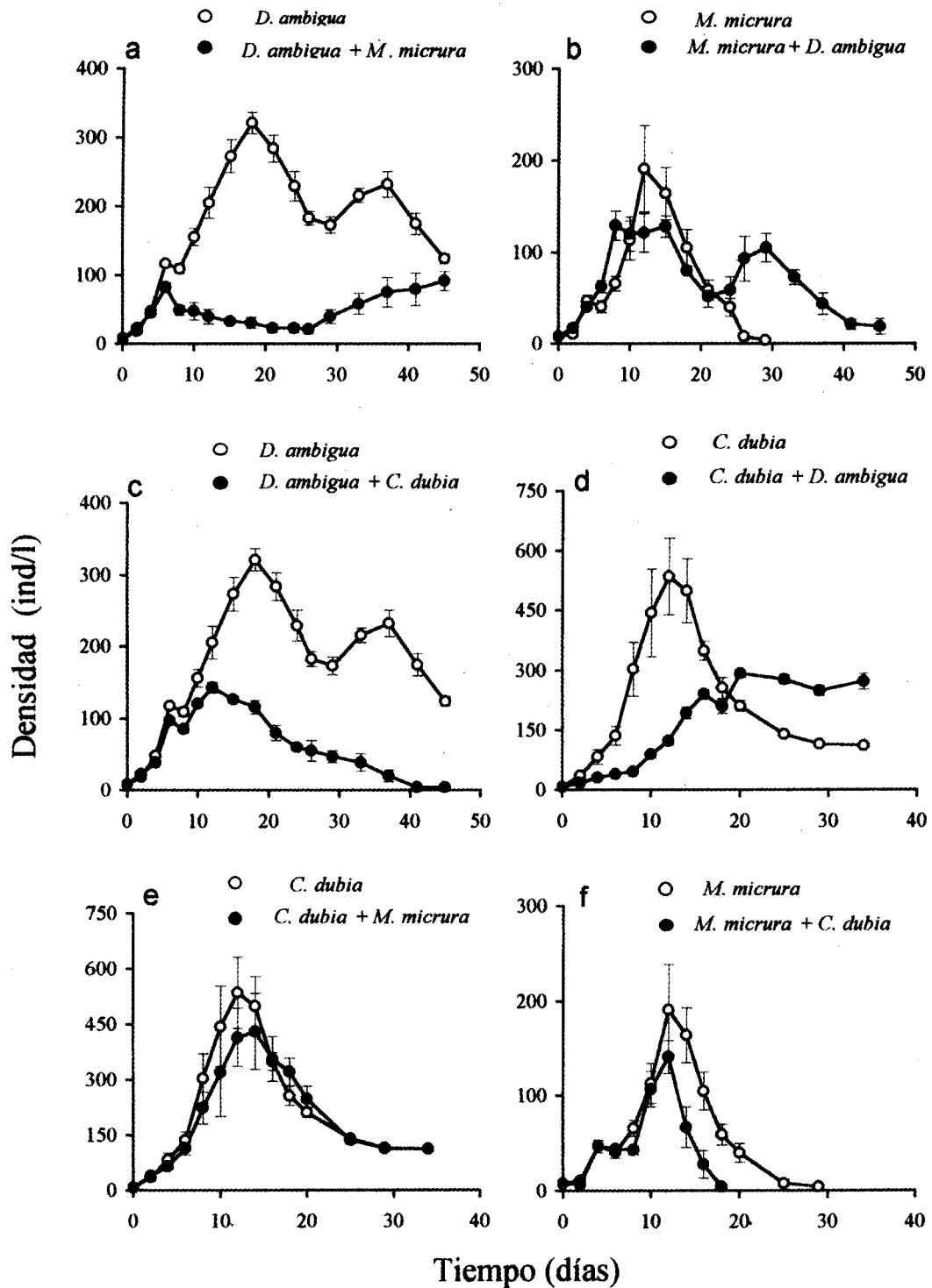
Fig. 2. Experimentos pareados: dinámicas poblacionales de los cladóceros Moina micrura , Ceriodaphnia dubia y Daphnia ambigua en condiciones de aislamiento (círculo abierto) y en coexistencia con otra especie (círculo cerrado). Todos los puntos presentan 1 EE (N = 3), con excepción del último punto de las curvas 2c y 2f.
