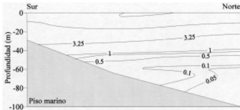
Fig. 11: Sección transversal Sur-Norte ( 70^{\circ}27'10'' ) de oxígeno disuelto en la columna de agua de la bahía Mejillones. Concentración de oxígeno en \text{mL L}^{-1} .
